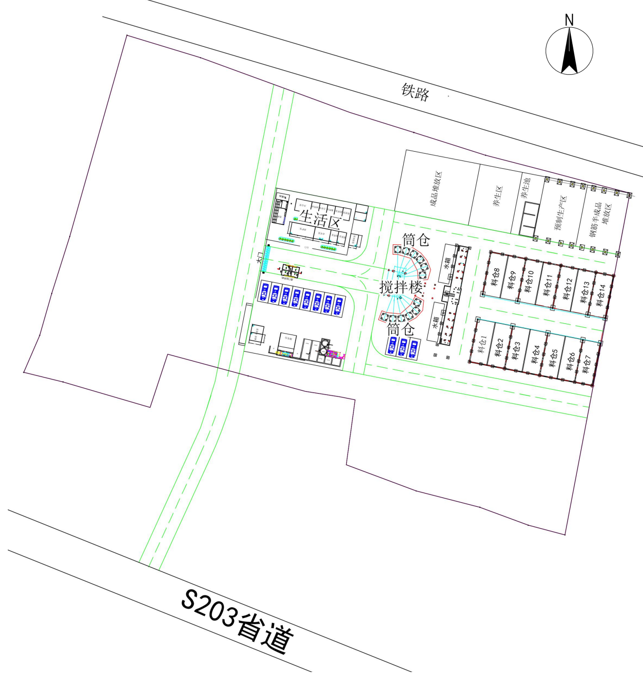
附图 4：平面布置图
