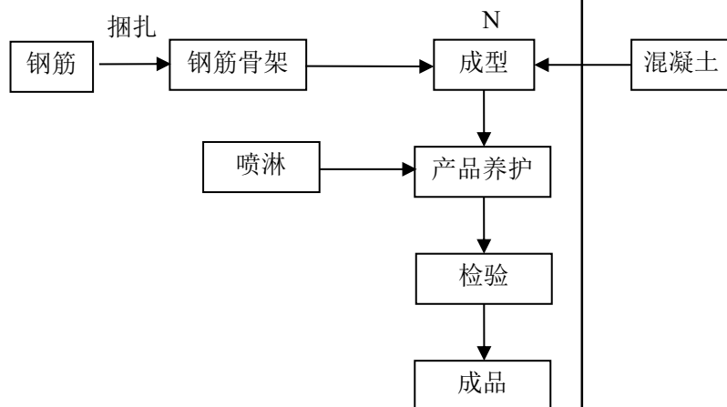
图 2-4 项目预制件工艺流程图及产排污环节示意图
